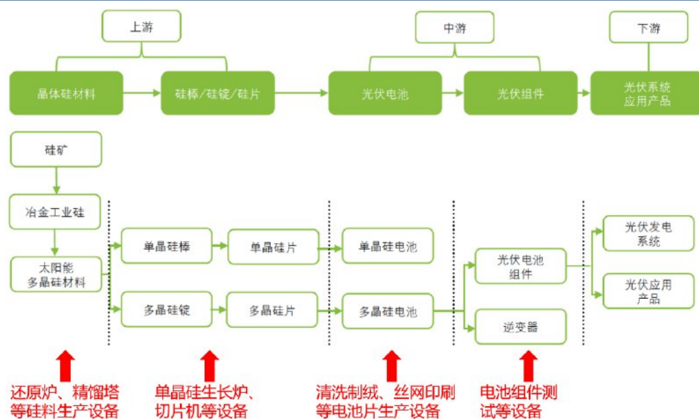
图表82：光伏发电系统生产流程与相关设备一览
