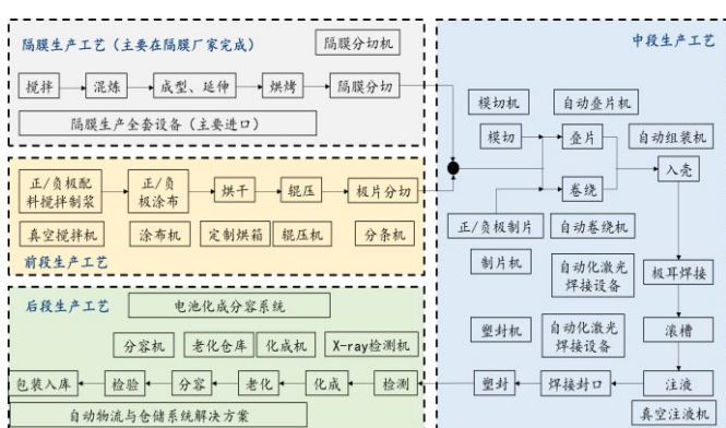
图表85：动力锂离子电池生产工艺全流程
