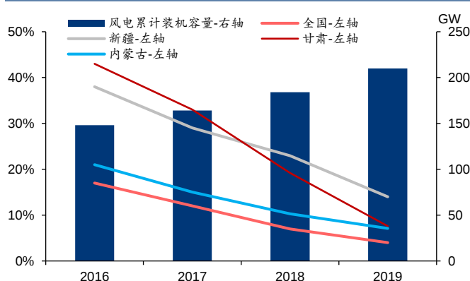
图表70：全国弃风率情况
