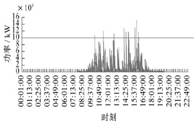
图表72：多云情况下光伏电站的输出功率波动量（1min 级别）
