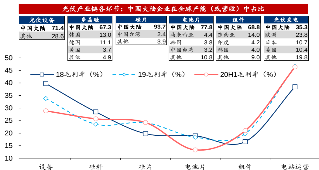
图6：中国已在光伏产业链“微笑曲线”中占据有利位置
