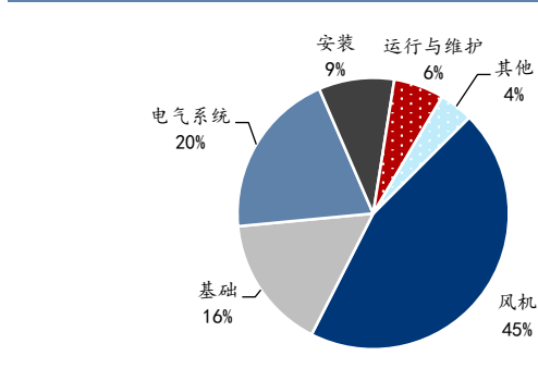
图表 64： 21 年海上风电投资约为 15000-17000 元/kW
