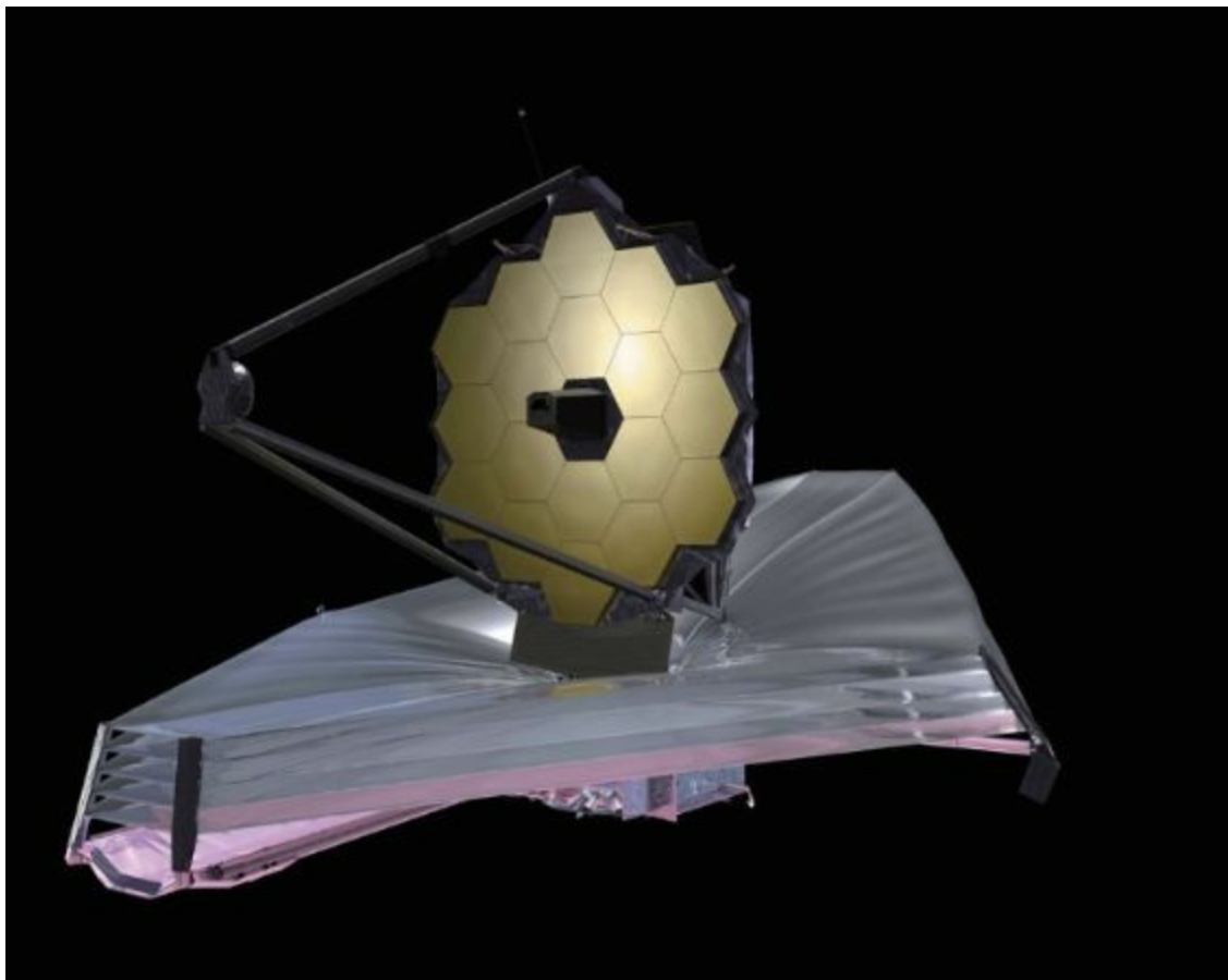
▲图5.4 詹姆斯·韦伯空间望远镜效果图
