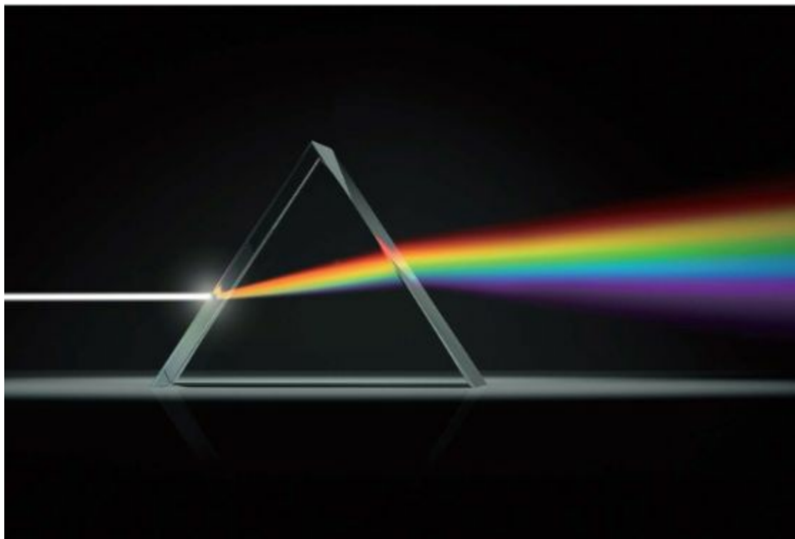
▲图5.3 光的色散
