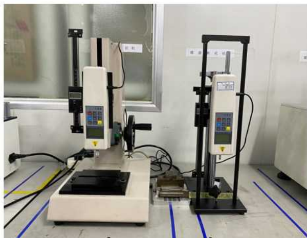
推拉力试验机 螺旋测试机
